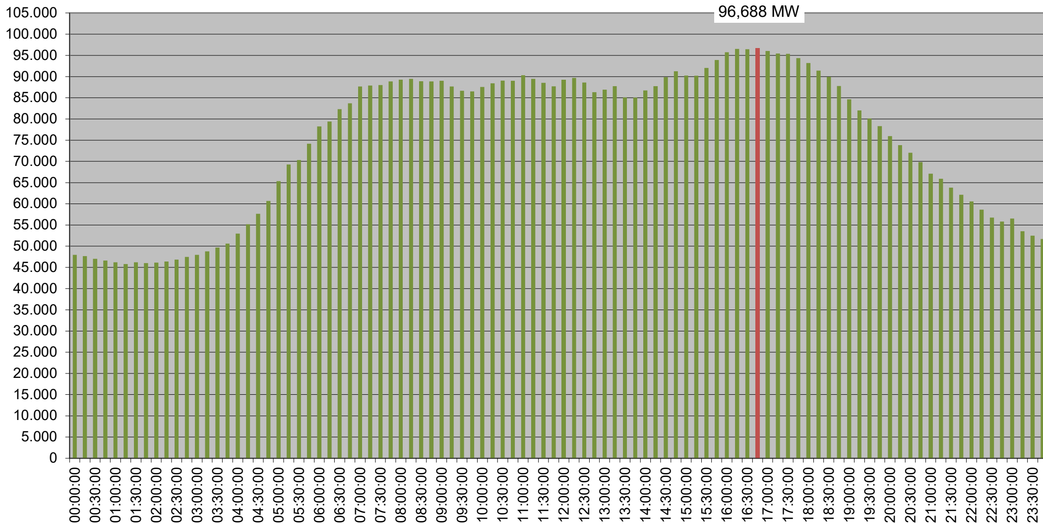
Verlauf der Netzlast HS/MS-Ebene am Höchstlasttag - 20.01.2022
