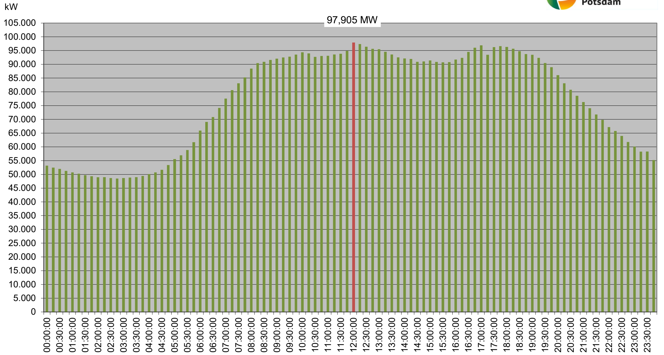
Verlauf der Netzlast MS-Ebene am Höchstlasttag - 11.01.2022
