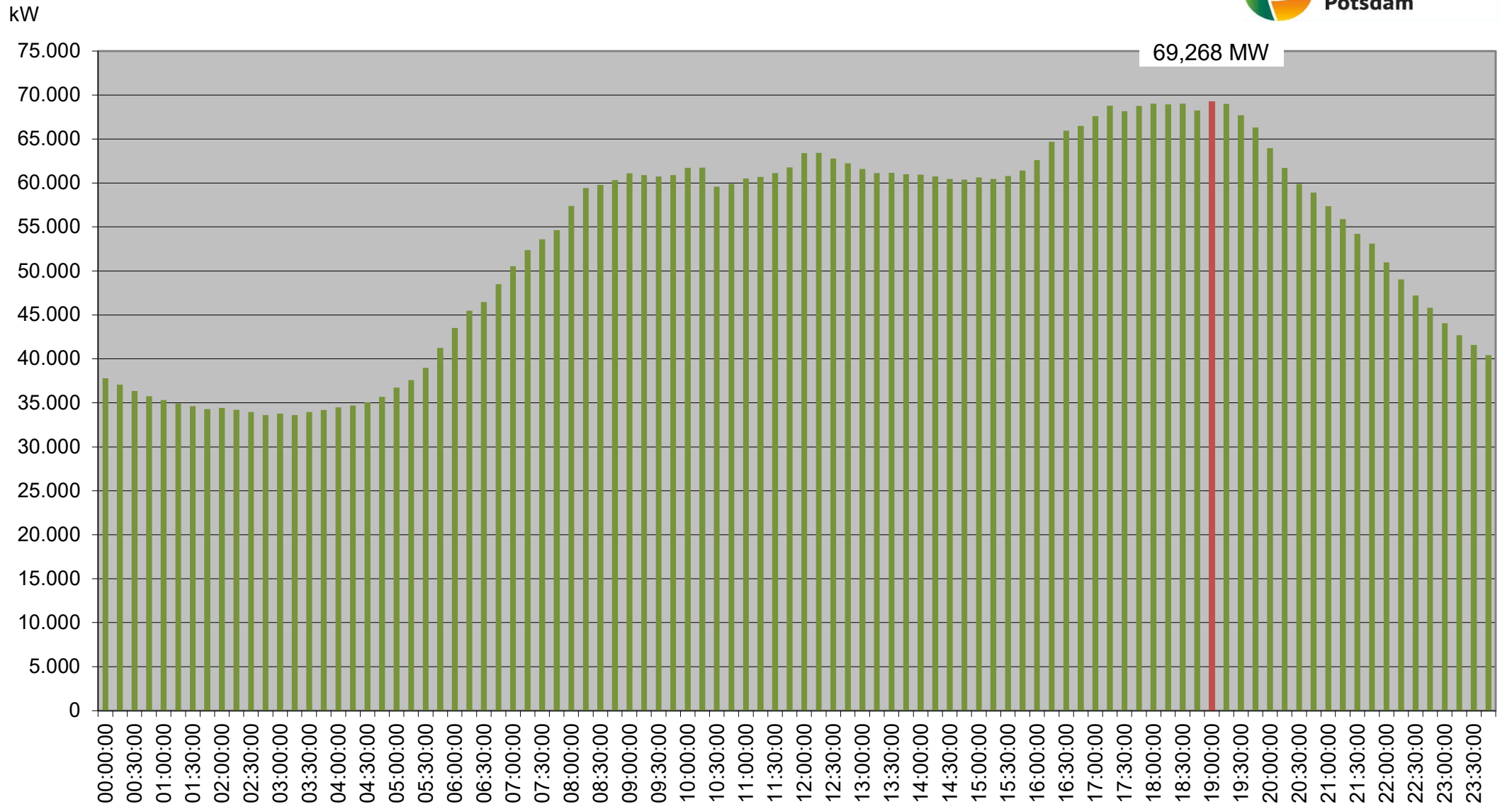
Verlauf der Netzlast MS/NS-Ebene am Höchstlasttag - 14.12.2022
